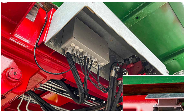
Die Hydac-Lenkung besteht aus einer separaten Steuerbox, einem Load-sensing-Block und einem kleinen Inertialsensor.
