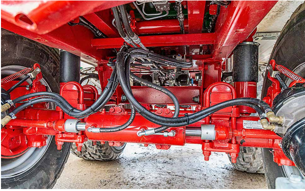
Die elektro-hydraulische Zwangslenkung erfordert Sensoren zur Geschwindigkeits-, Fahrtrichtungs- und Lenkerkennung.
