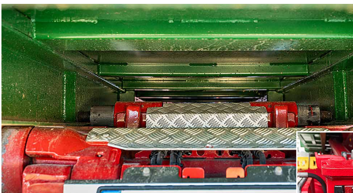
Vorne zeigen gut einsehbare LED den Zustand der Achsabstützung und Containerverriegelung (links) an.
